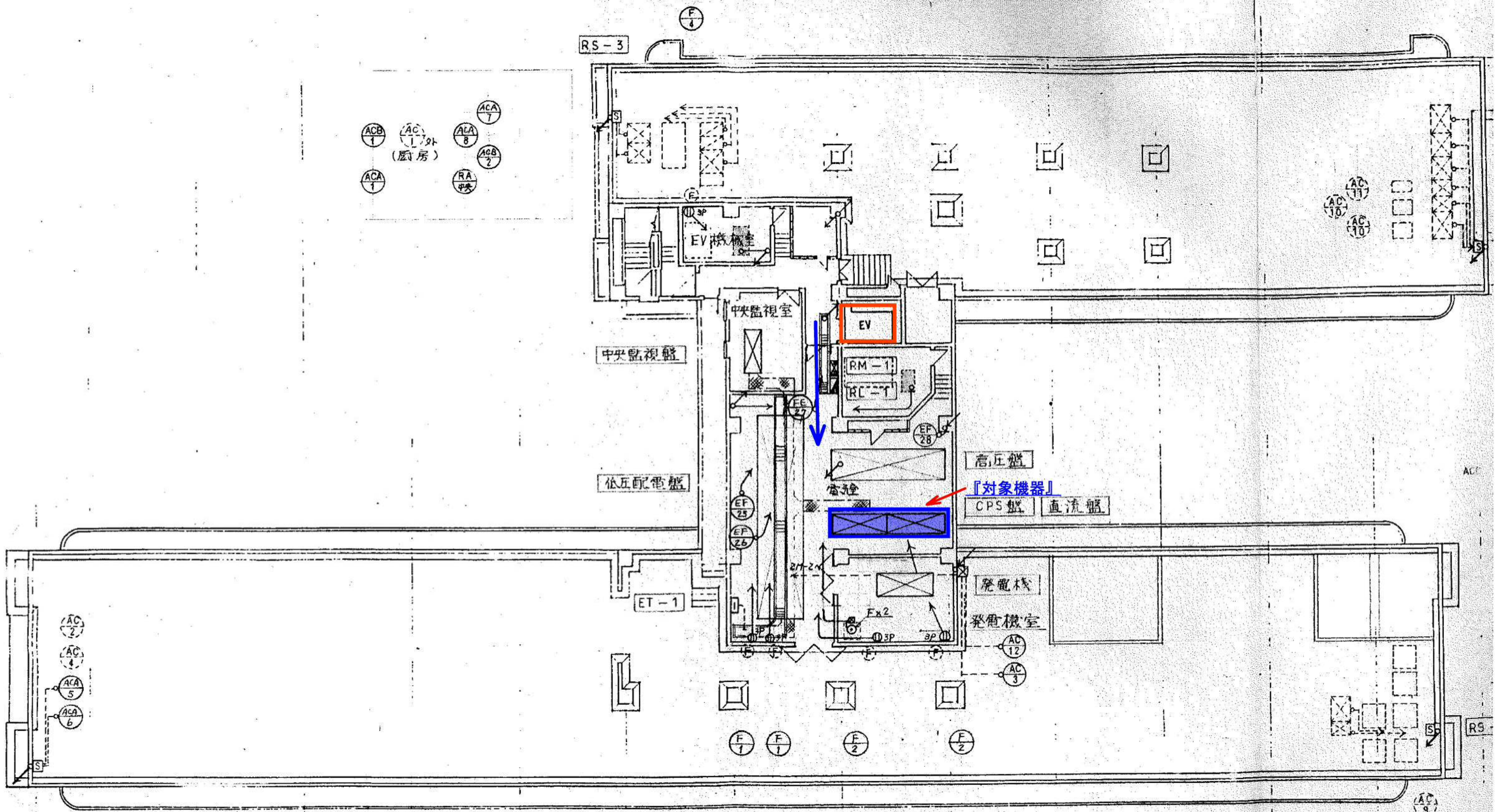
PH1 階配線図 1:200
