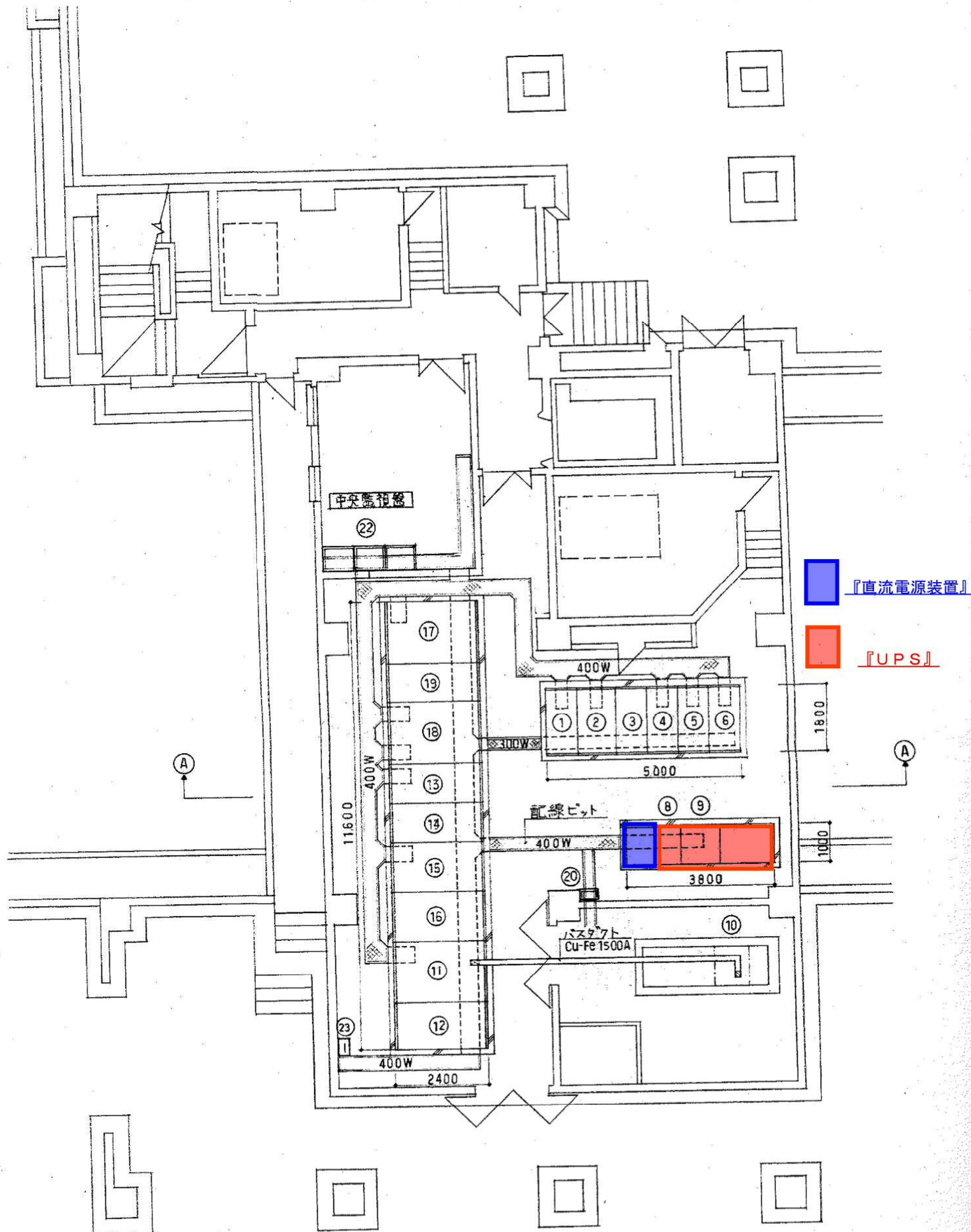
電気室平面図 S=1/100
